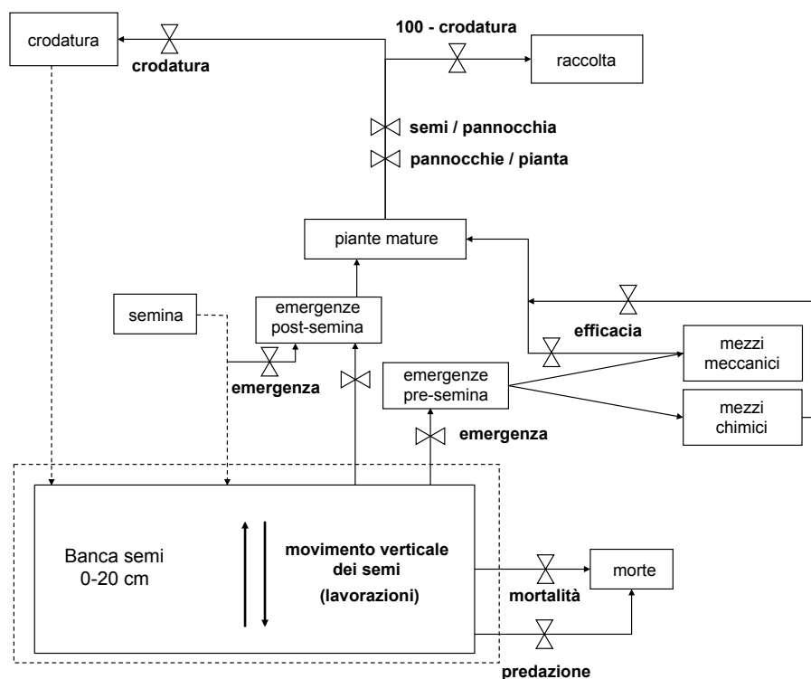
Figura 2. Rappresentazione simbolica della struttura del modello, con indicazione delle variabili di stato (rettangoli), dei flussi (frecche) e dei tassi (X) che regolano i flussi (da Vidotto e Ferrero, 2005, modificato).
