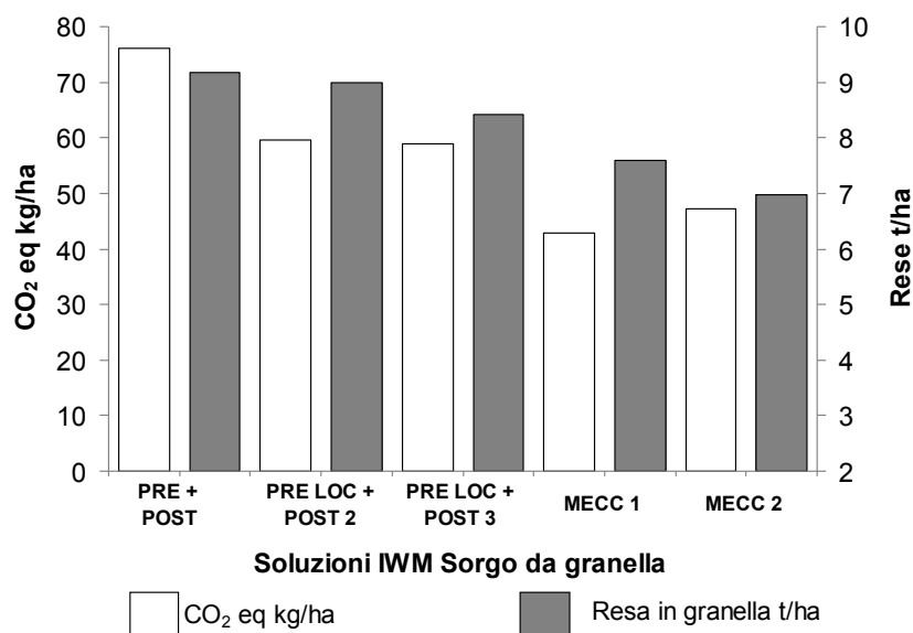
Figura 6. Carbon Footprint espresso in kg/ha di CO 2 equivalente e rese in t/ha in colture di sorgho da granella coltivati in 5 tesi IWM a confronto.
